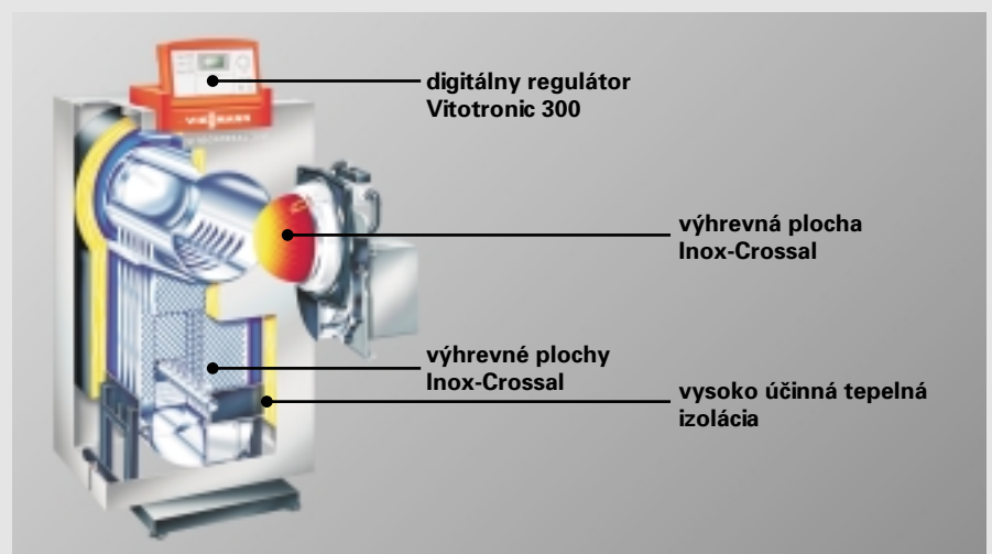
Vysoko hodnotný nerezový kotol Vitocrossal 300
