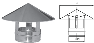
010 Hlavica proti dažďu
