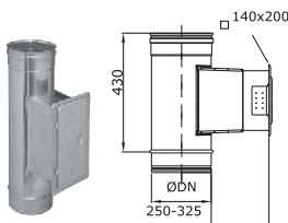
521 Revízny kus s dvierkami
