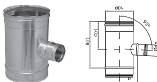
312 Redukčný T – kus 93°
