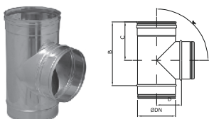
31A T – kus 93°
